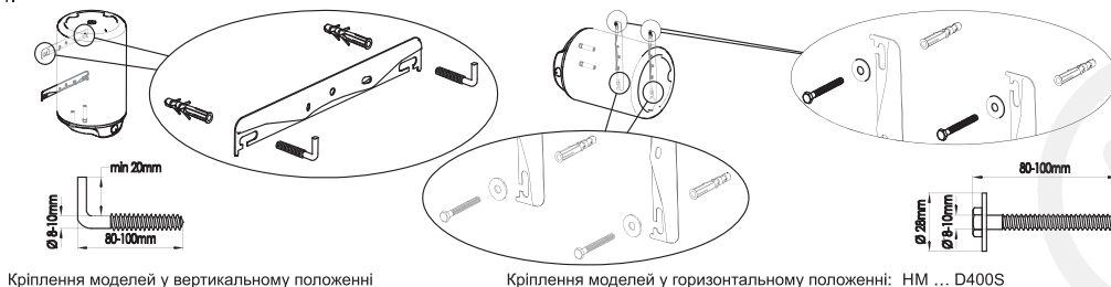
Рисунок 4. Кріплення ЕВАД до стіни
