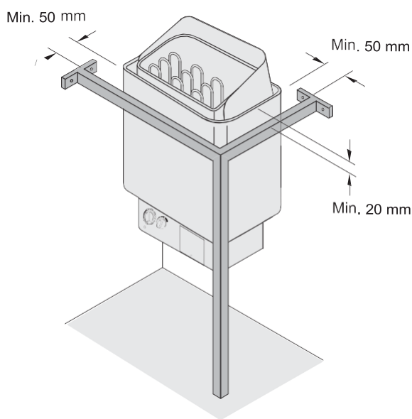
Fig. 4. Safety railing Рис. 4. Защитное ограждение
