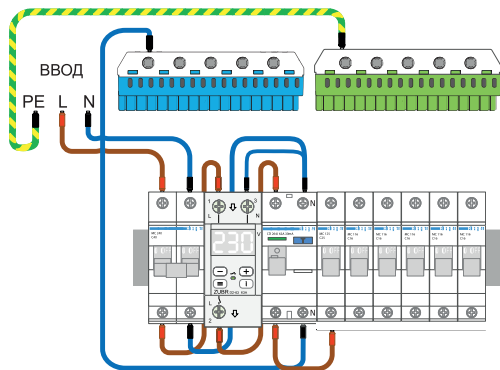
Схема 2. Вариант монтажной схемы D2
