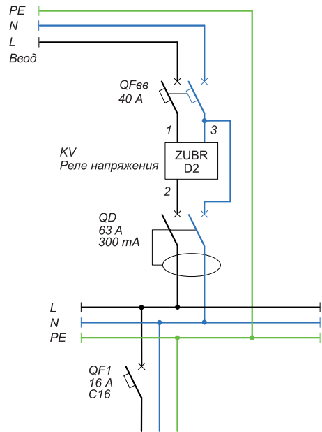
Схема 1. Вариант электрической схемы D2
