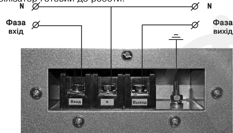
Мал.3. Схема підключення стабілізатора
