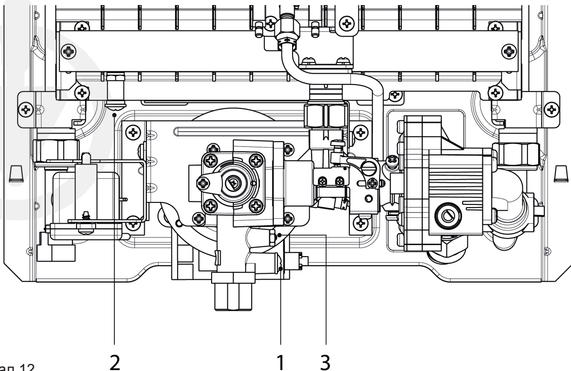
Мал.12
