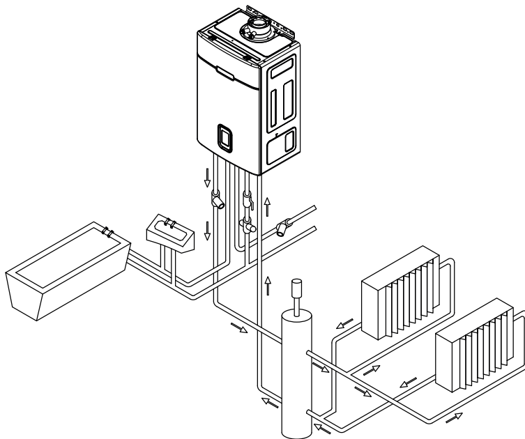
Рисунок 7. Приклад монтажу системи опалення та ГВП.
