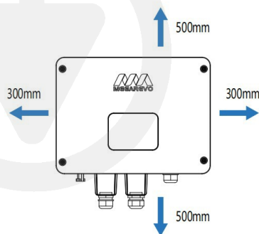
Мал. 4-2 Монтаж інвертора
