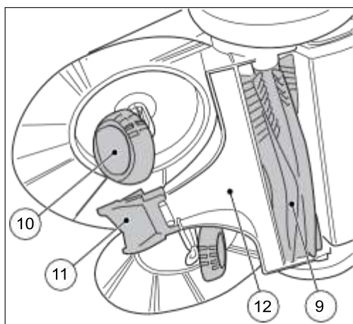
Мал. 2: Огляд компонентів 2
