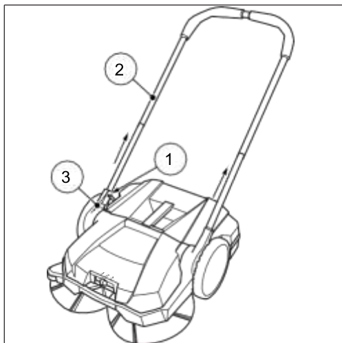
Мал. 12: Монтаж телескопічної ручки
