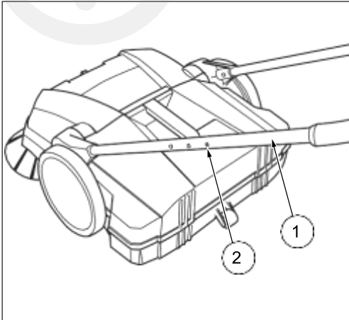
Рис. 9: Регулювання висоти телескопічної ручки
