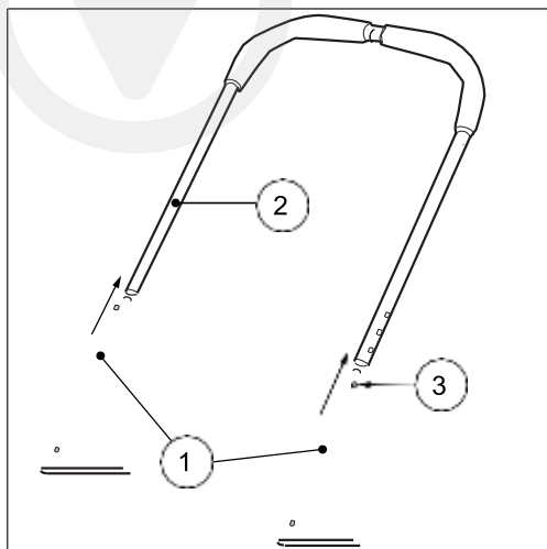
Мал. 7: Монтаж телескопічної ручки
