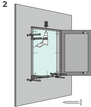
крёпёж короба
