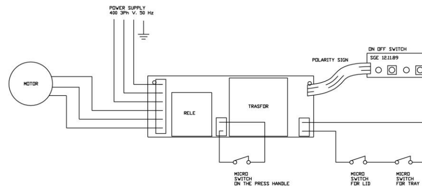
Мал. 21 – Схема трифазної електричної системи
