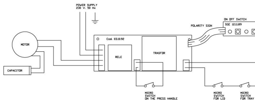
Мал. 21А - Схема однофазної електричної системи 230 В
