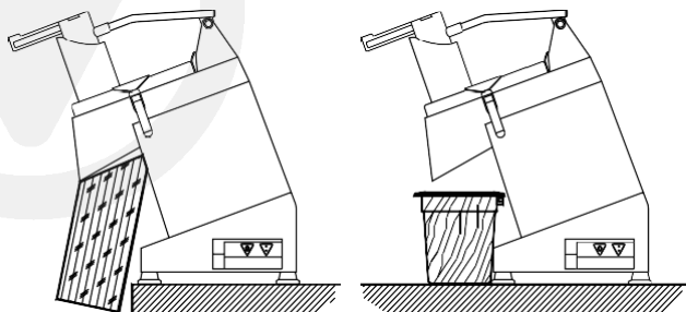
Мал. 4 – Розташування каналу або ємності, що дозволяє здійснити запуск пристрою
