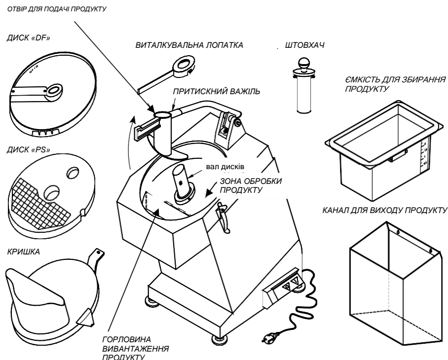
Мал. 28 – Видяг пристрою, розібраного для очищення
