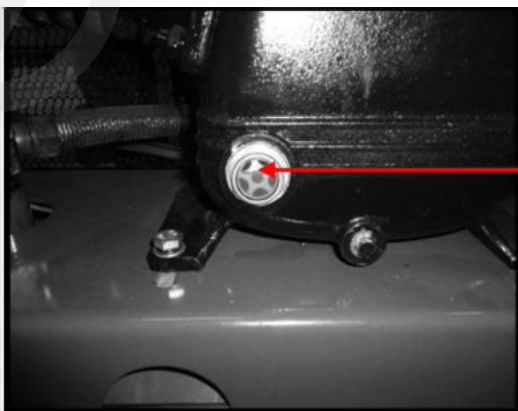
Рівень оливи
